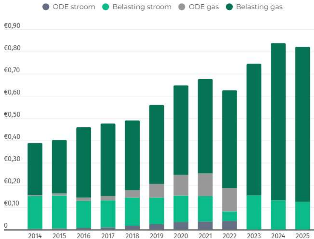
Overheidsheffingen per kWh stroom en m 3 gas
